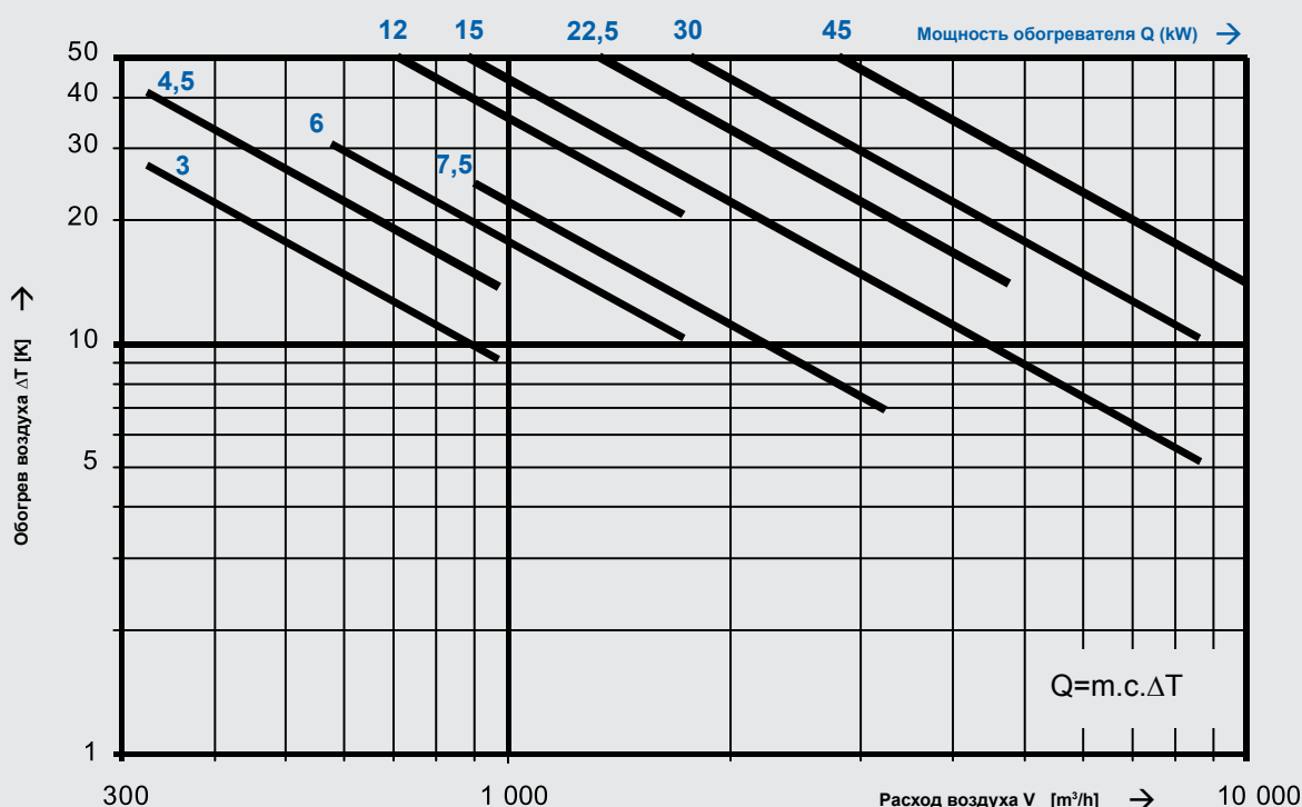
Рис. 4 – увеличение температуры воздуха на обогревателе в зависимости от расхода
