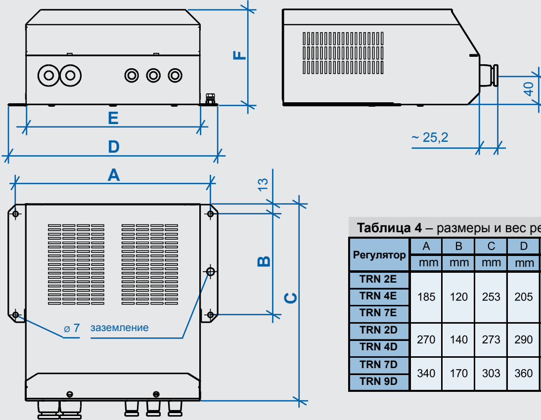
Рис. 15 – размеры и вес регуляторов TRN
