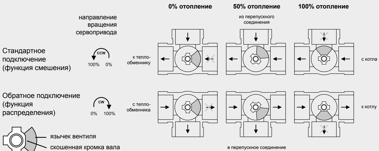
Рис. 11 – Функции трехходового вентиля
