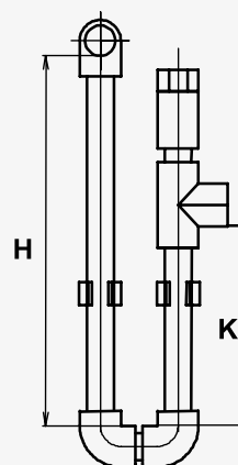
Рис. 5 – отвод конденсата
