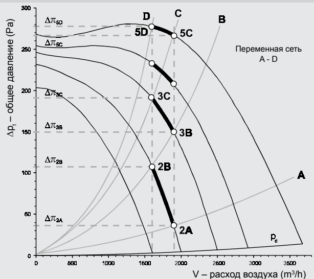
Рис. 4 – характеристика сети
