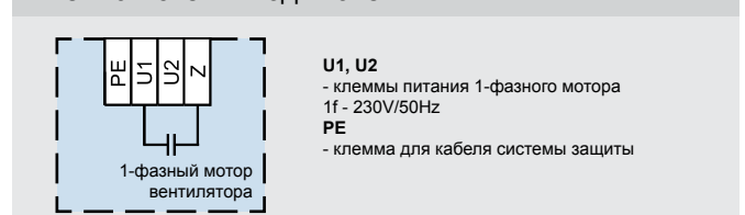
Рис. 10 - схемы подключения
