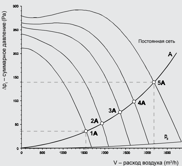
Рис. 2 – максимальный расход воздуха
