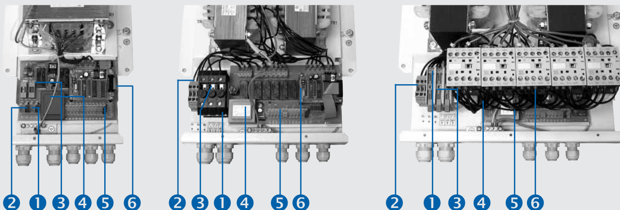
Рис. 17 – подключение регулятора
