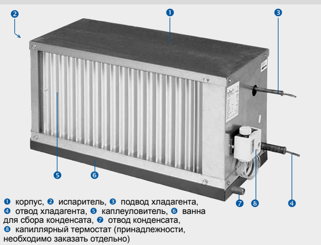
Рис. 1 - конструкция прямого охладителя
