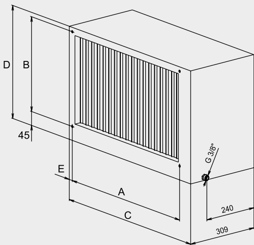
Рис. 4 - размеры каплеуловителей
